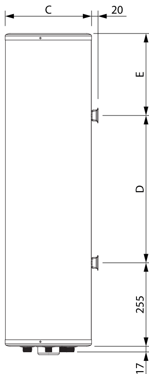
вид сбоку
