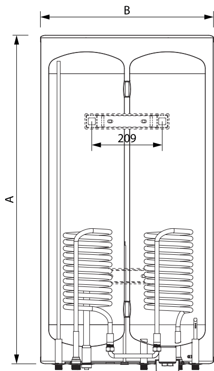
вид спереди в разрезе
