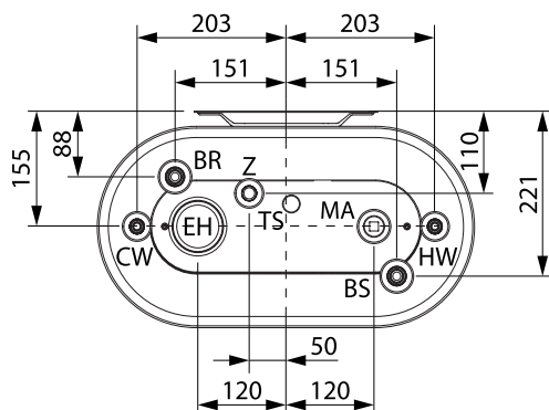
вид снизу
